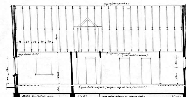
DOORSNEDE A-B.
