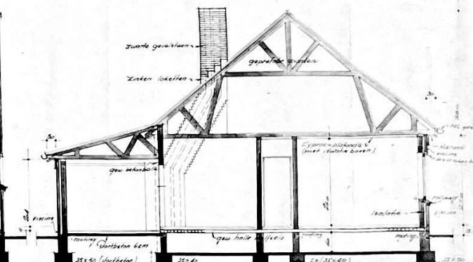
DOORSNEDE C-D.
