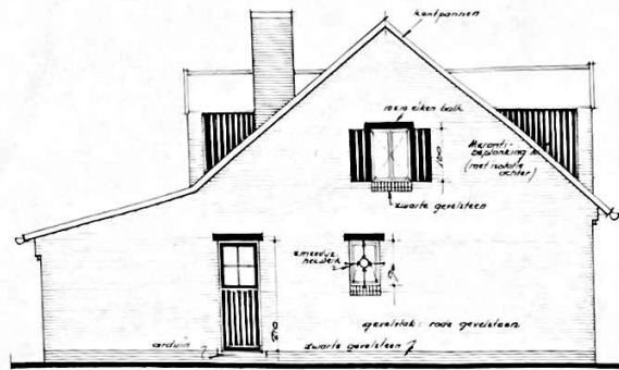
ACHTERGEVEL.
