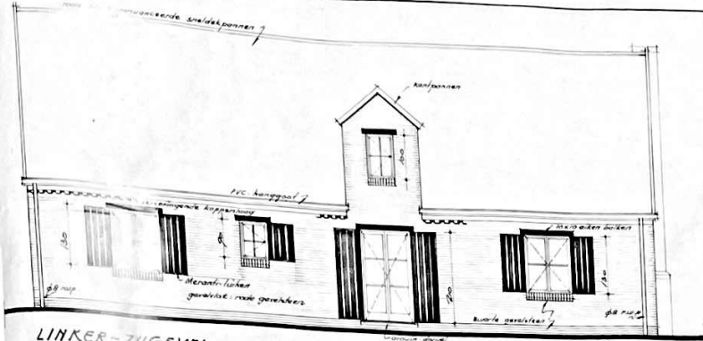
LINKER-ZIGEVEL.
