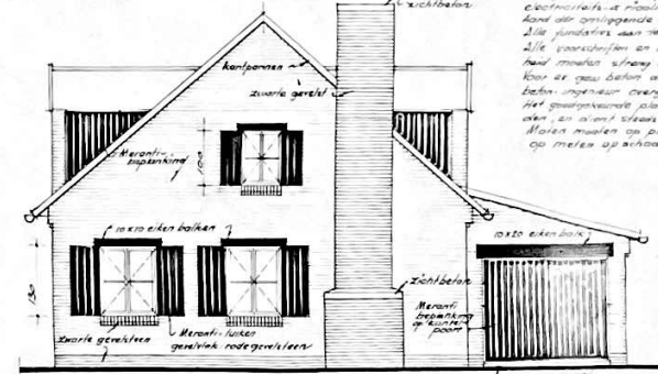
VOORGEVEL.
